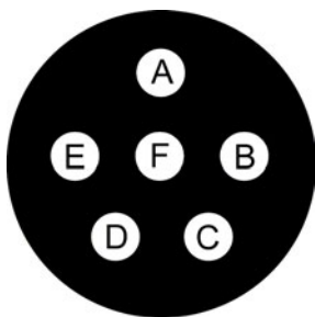
MIL Stecker 06 10 98SN
